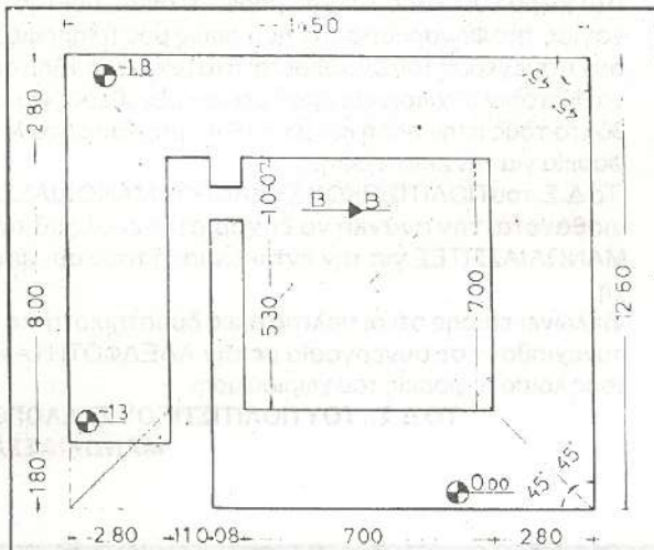
Σχ. 1. Κάτοψη της πυραμίδας του Ελληνικού.
